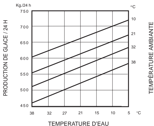
MACHINES À REFROIDISSEMENT PAR AIR
