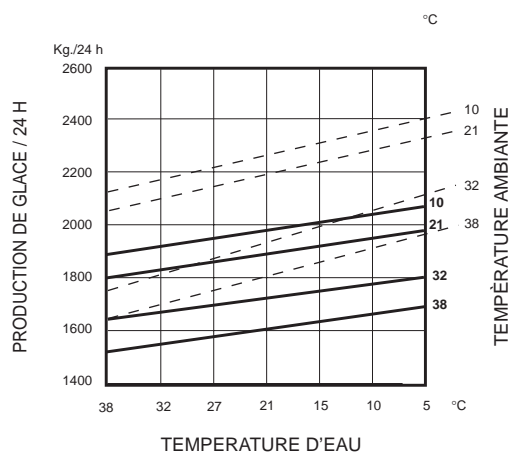
MACHINES À REFROIDISSEMENT PAR AIR
