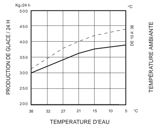
MACHINES À REFROIDISSEMENT PAR EAU
