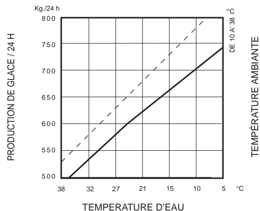
MACHINES À REFROIDISSEMENT PAR EAU
